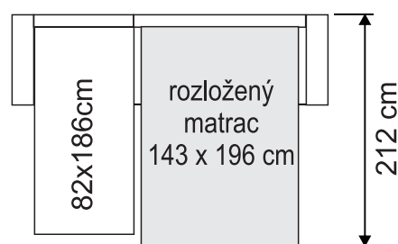
súprava DU-3SR140-B :
